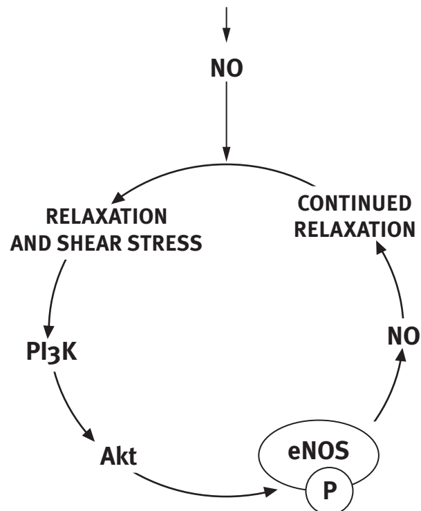
FIGURE 3 : Mécanisme cellulaire du maintien de l'érection : rôle prépondérant du NO (emprunté à Arthur Burnett).
