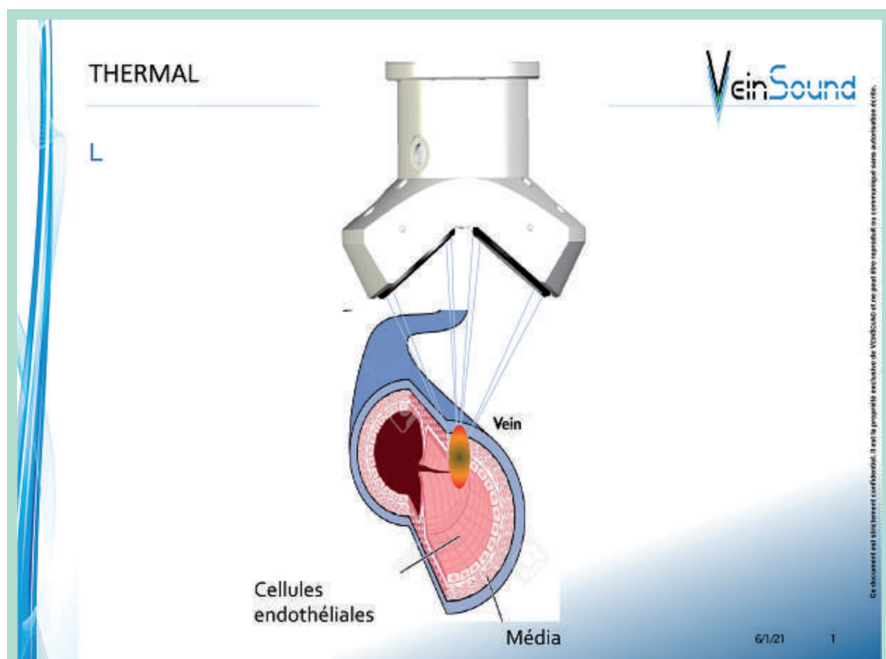
FIGURE 1 : Principe des HIFU.
