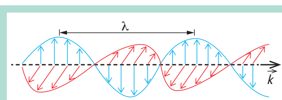
FIGURE 3 : Onde électromagnétique.
