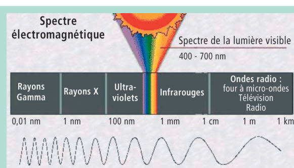
FIGURE 4 : Spectre des ondes électromagnétiques.
