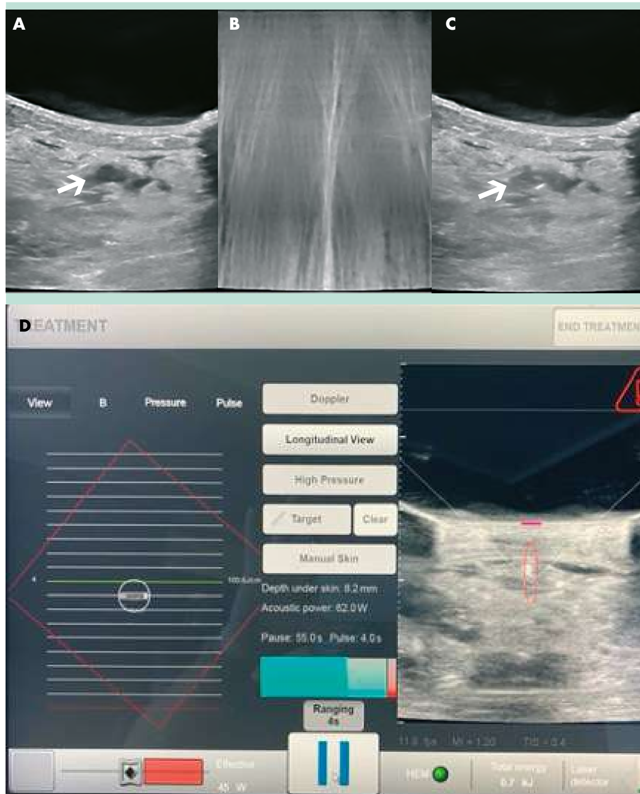
FIGURE 2: Procédure HIFU.
