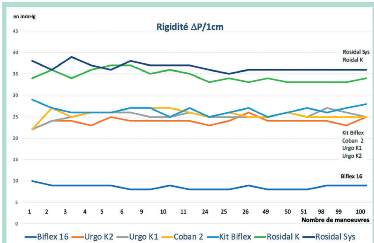
FIGURE 3 : Comparaison de l'évolution de la rigidité pour Urgo K1, Urgo K2, Rosidal K et Rosidal Sys.
