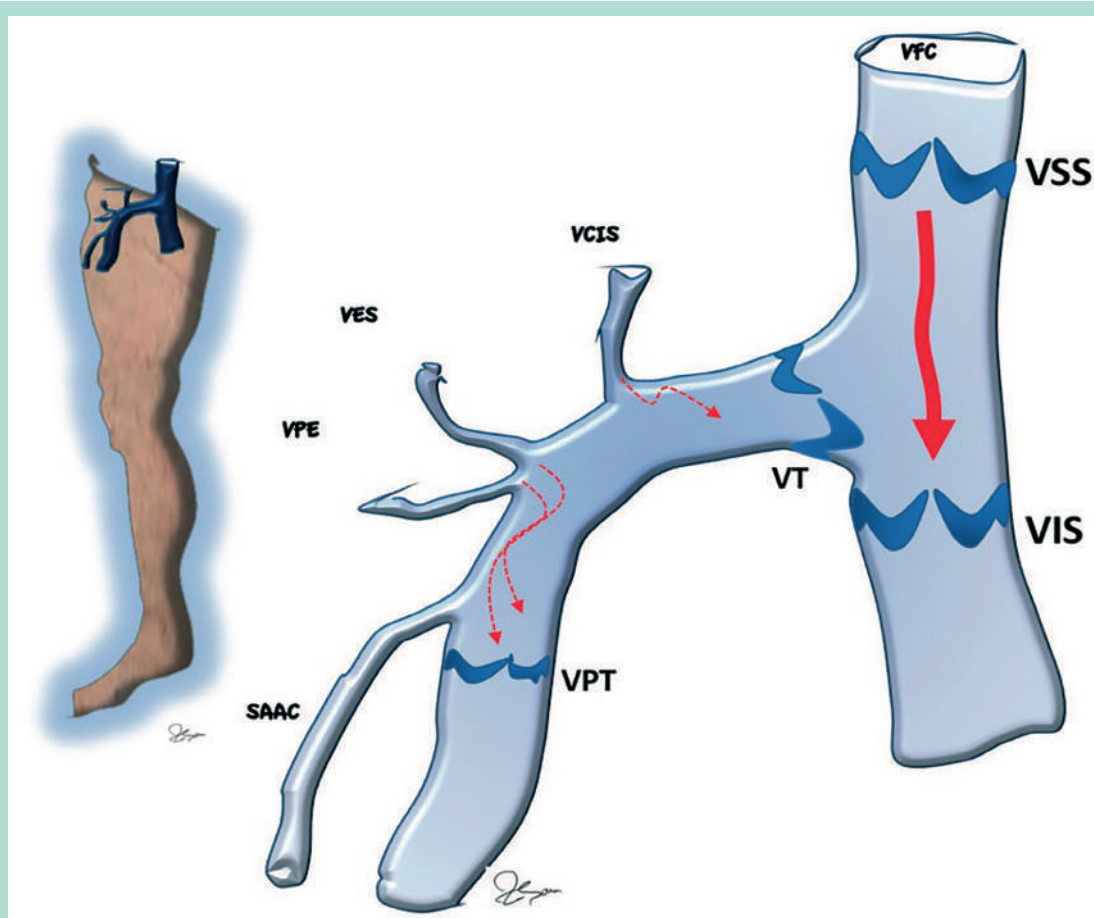
FIGURE 7 : Lors de la diastole musculaire. Valves pré-terminale et terminale fermées. Elles s'opposent au flux gravitaire des veines circonflexe superficiel VCS, Veine épigastrique superficielle (VES). Fragmentation de la colonne de pression de la veine fémorale par la valve supra-saphénique (VSS) et la valve infra-saphénique (VIS). Schéma S. Zerrouk.
