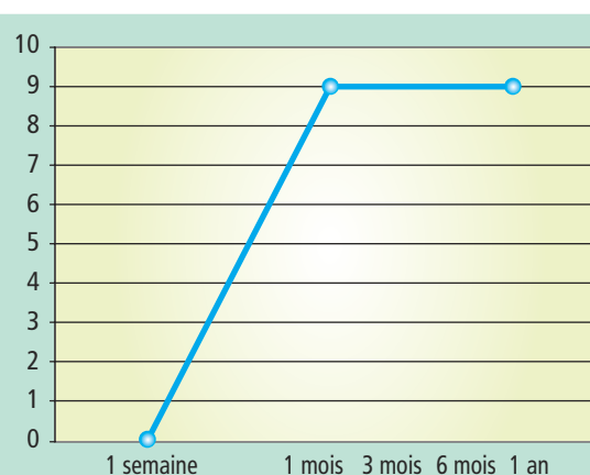
FIGURE 6 : Efficacité de la sclérose sur les ectasies. La taille des ectasies (2,72 mm de diamètre en moyenne) n'a pas été un critère de leur sclérose par le laser.
