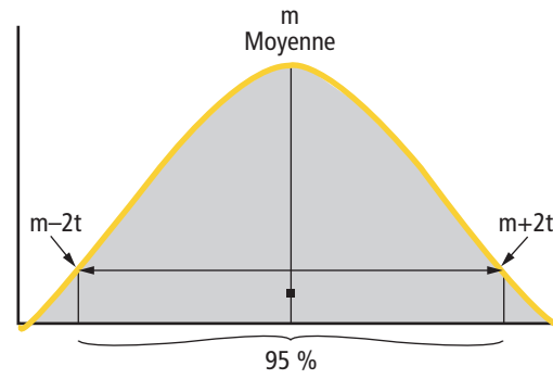
FIGURE 5 : Distribution de la population en fonction de la moyenne m et de l'écart-type t .
