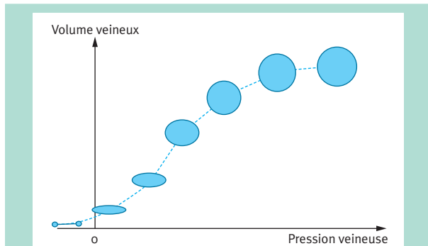
FIGURE 2 : Évolutions de la forme de la section veineuse et du volume contenu dans la veine, en fonction de la pression interne (d'après [4]).
