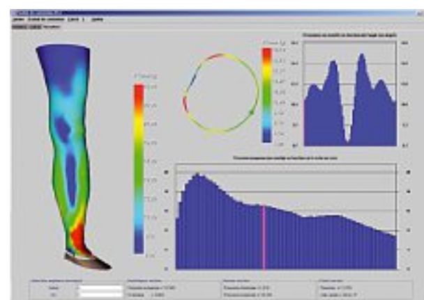
FIGURE 4 : Logiciel des pressions (LP) : capture d'écran du LP. À gauche : cartographie 3D des pressions appliquées à la peau. À droite en haut : cartographie 2D sur coupe de mollet et profil de pression sur coupe. À droite en bas : profil des pressions moyennes par cote, du cou de pied (à gauche) vers la cuisse.
