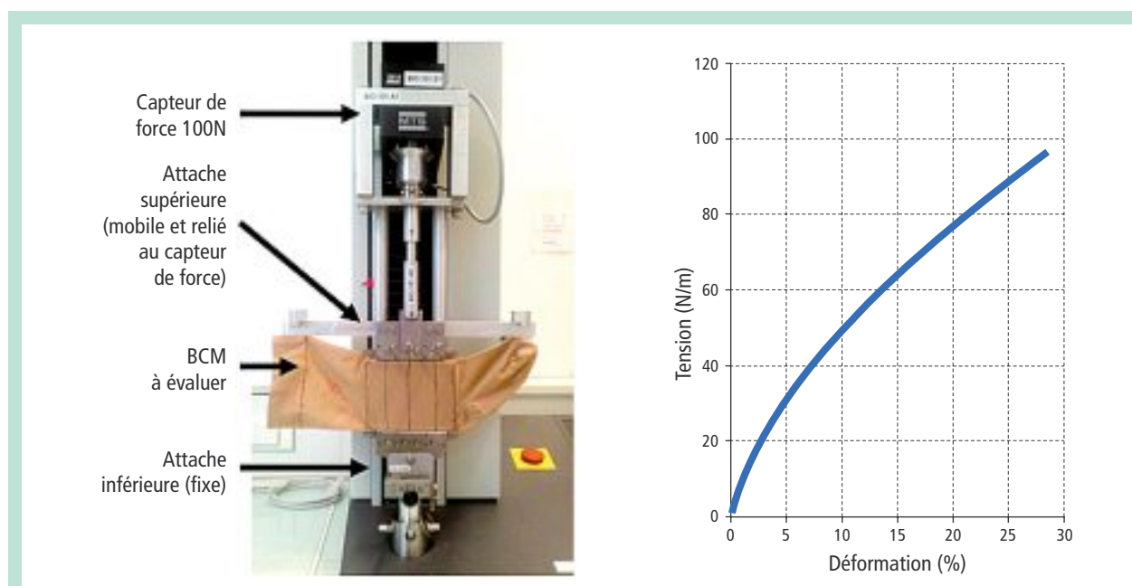
FIGURE 2 : Caractérisation du comportement mécanique d'un BCM. À gauche : banc expérimental. Dynamomètre MTS 200/M avec capteur de force 100N et BCM en cours de mesure. À droite: courbe tension-déformation (exemple de résultat). La courbe bleue représente la tension (en N/m, en ordonnée) en fonction de la déformation (en %, en abscisse) du BCM mesuré.
