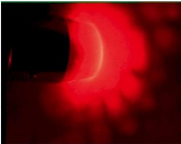
Fig. 1. – Réseau réticulaire
