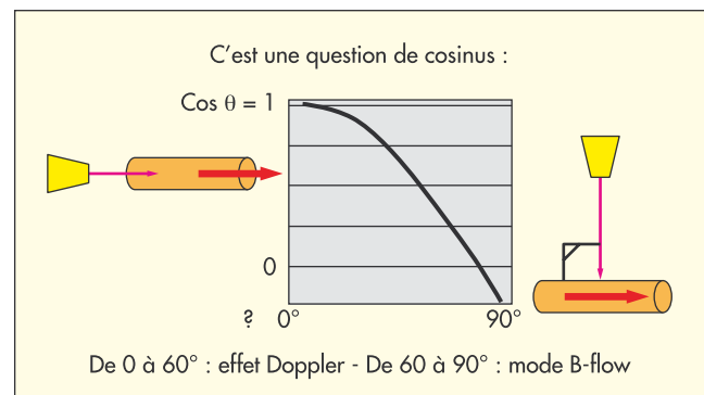
Schéma 4. – Complémentarité d'angle du faisceau incident d'ultrasons entre le mode B-flow et l'effet Doppler
