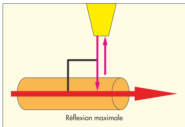
Schéma 1. – La réflexion est maximale si le faisceau incident est perpendiculaire à l'interface
