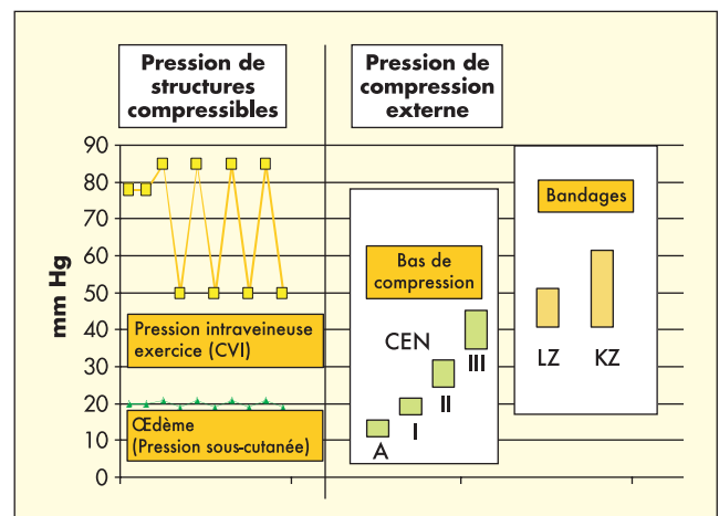
Figure 3. – Dans la moitié gauche de la Figure, les valeurs de pression sont représentées de façon exemplaire comme elles peuvent être mesurées dans la structure compressible de la peau dans le cas d'un œdème respectif dans une veine de la partie distale de la jambe d'un patient porteur d'une insuffisance veineuse chronique de grade moyen (CVI). Dans la moitié droite de la figure, ces valeurs de pression sont restituées schématiquement telles qu'elles seraient exercées par des bas de compression classe 1 à 3 correspondant à la norme européenne (CEN), respectivement par des bandages à allongement long (LZ) et à allongement court (KZ), qui furent appliqués chaque fois avec une pression de repos de 40 mm Hg. On note que seul le bandage à allongement court produit à la marche des pics de pression qui dépassent de façon intermittente les valeurs de pression intraveineuse. En comparaison, les bas de compression classe 2 et 3 sont capables de comprimer un œdème chez un sujet en situation debout mais pas les veines jambières
