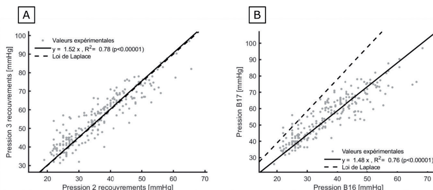
FIGURE 2 : A - Pression appliquée par un bandage à 3 recouvrements en fonction de la pression exercée par un bandage à 2 recouvrements ; B - Pression appliquée par la bande B17 en fonction de la pression appliquée par la B16.
