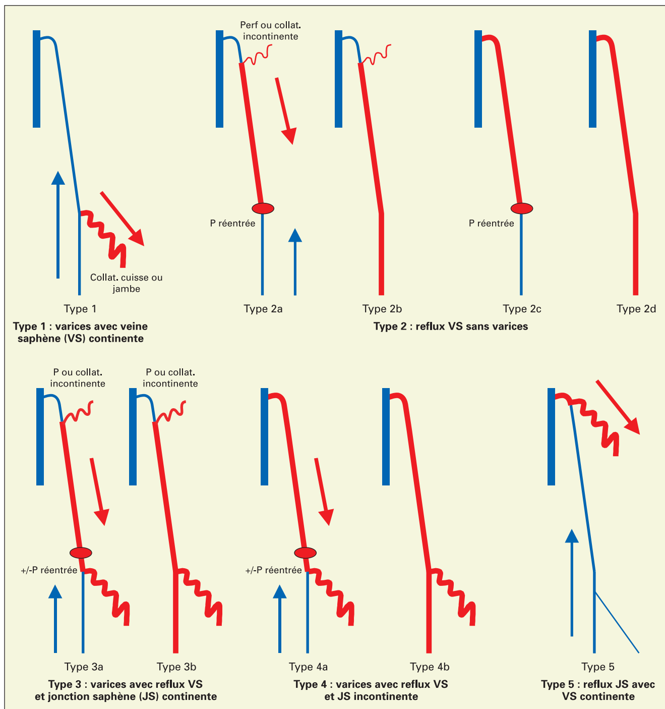
Fig. 1. – Typologie écho-Doppler
