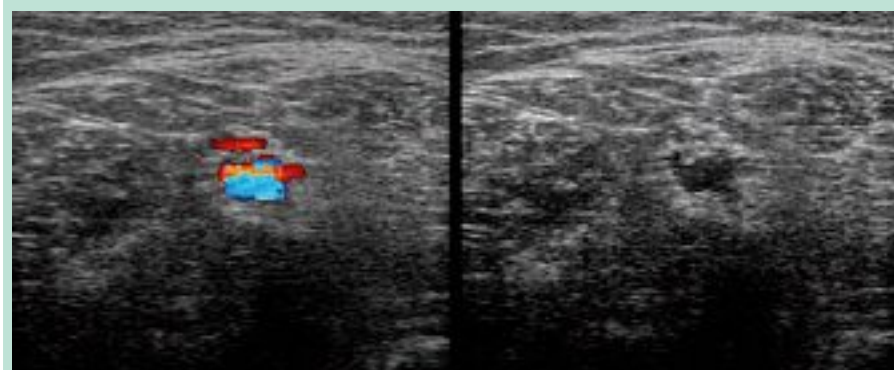
FIGURE 11 : La varice du nerf sciatique (le reflux est montré par le Doppler couleur), en général très discrète, pénètre le nerf et passe à travers ses fibres nerveuses ou son périnévrion avec une image échographique très particulière en « cible ».
