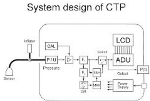
Principe de détection du Professeur Blazek
