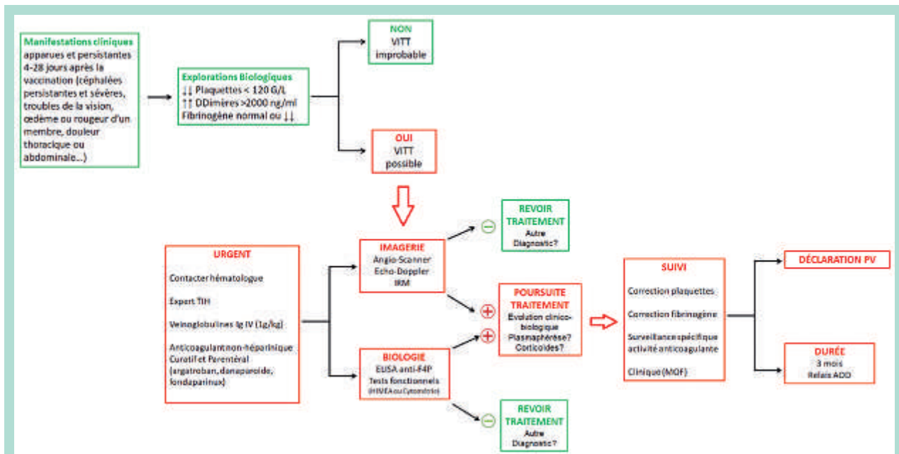
FIGURE 3 : Algorithme décisionnel en cas de suspicion de VIT [d'après 52-55].
