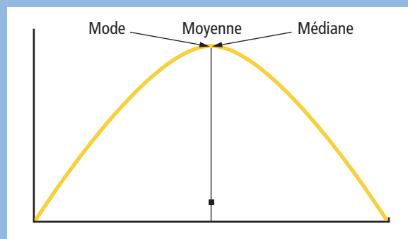
FIGURE 1 : Distribution symétrique.
