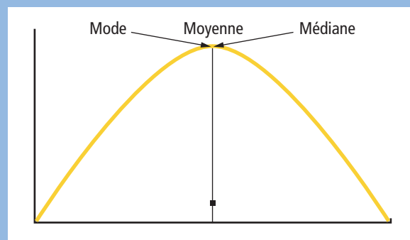
FIGURE 1 : Distribution symétrique.
