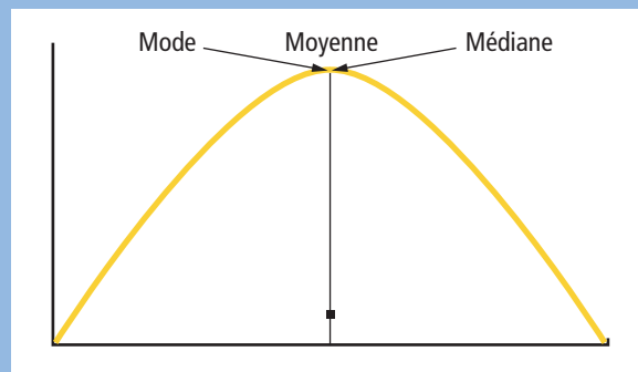
FIGURE 1 : Distribution symétrique.
