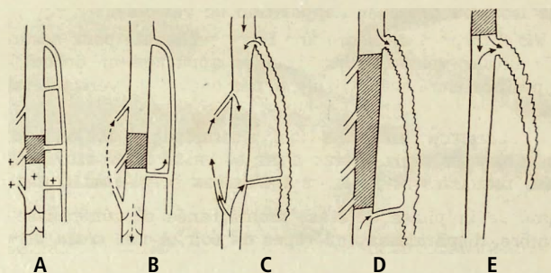
Schéma des altérations hydrauliques après oblitération profonde
