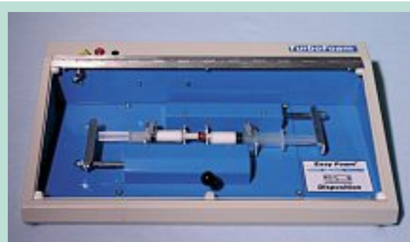
FIGURE 6 : Machine standardisant le va-et-vient pour la fabrication de la mousse, 2004
