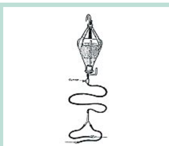
FIGURE 4 : Remplissage par gravité ressemblant au système « piuvre ».
