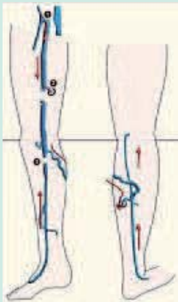
FIGURE 3 : Schéma de la cartographie veineuse droite après la cure CHIVA. 1 Crossotomie avec suture fémorale latérale. 2 Ligature résection à mi cuisse sous la perforante fémorale. 3 Ligature sous gonale sous lacommunicante. (Le geste a été complété par des phlébectomies des varices distales).
