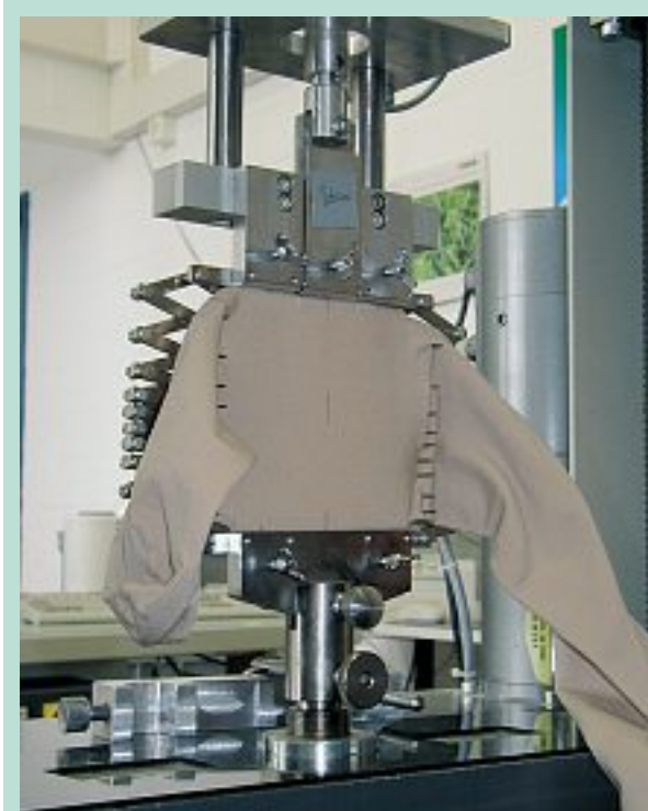
FIGURE 8 : Dynamomètre, instrument permettant d'obtenir la courbe caractéristique des matériaux force = f(\text{allongement}) .
