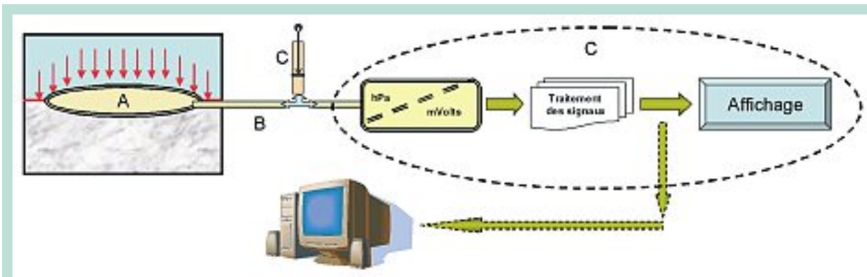
FIGURE 9 : Principe de mesure de pression d'interface in-situ.
