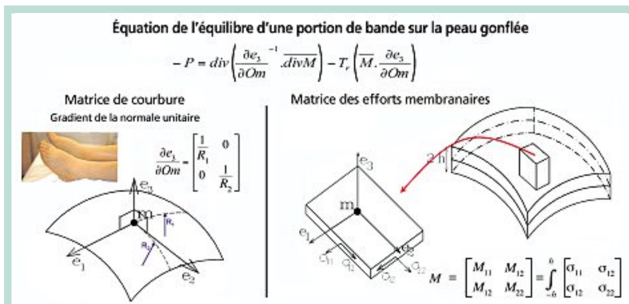
FIGURE 6 : Formulation complète de la loi de Laplace en version « 3D ».
