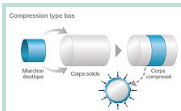
FIGURE 4 : Compression de type anneau élastique.
