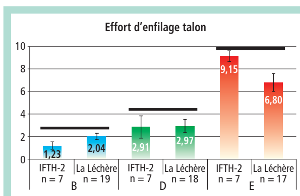
FIGURE 4 : Valeurs moyennes des efforts d'enfilage talon pour les populations IFTH (étude 2) et La Léchère complète. Une barre horizontale indique l'absence de différence significative selon le test de Mann-Whitney à 5 %.
