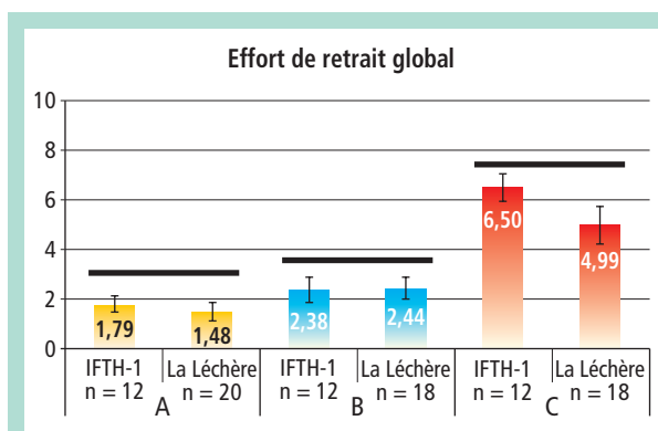
FIGURE 3 : Valeurs moyennes des efforts de retrait global pour les populations IFTH (étude 1) et La Léchère complète. Une barre horizontale indique l'absence de différence significative selon le test de Mann-Whitney à 5 %.
