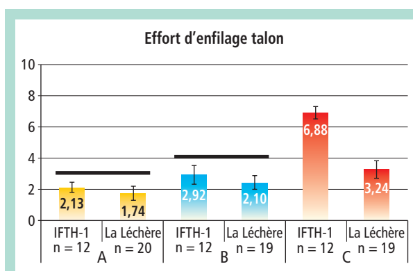
FIGURE 2 : Valeurs moyennes des efforts d'enfilage talon pour les populations IFTH (étude 1) et La Léchère complète. Une barre horizontale indique l'absence de différence significative selon le test de Mann-Whitney à 5 %.
