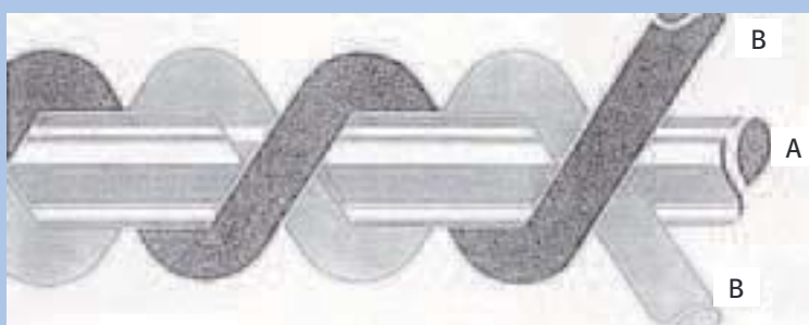
FIGURE 3 : SCHEMA DE PRINCEPE : A : âme élastique . B : fils de couverture.
