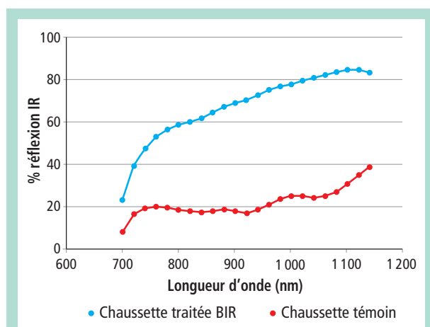
FIGURE 1 : Pourcentage de réflexion des infrarouges proches par : – une chaussette de compression noire standard (chaussette témoin, courbe rouge) – et une chaussette de compression noire traitée Coldblack® (chaussette traitée BIR, courbe bleue) lors des tests in vitro .
