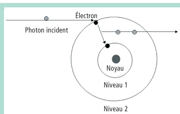
FIGURE 5 : Action du laser sur un atome.
