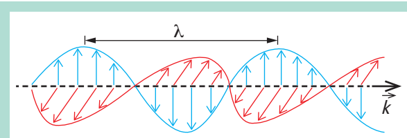
FIGURE 3 : Onde électromagnétique.
