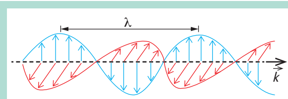
FIGURE 3 : Onde électromagnétique.
