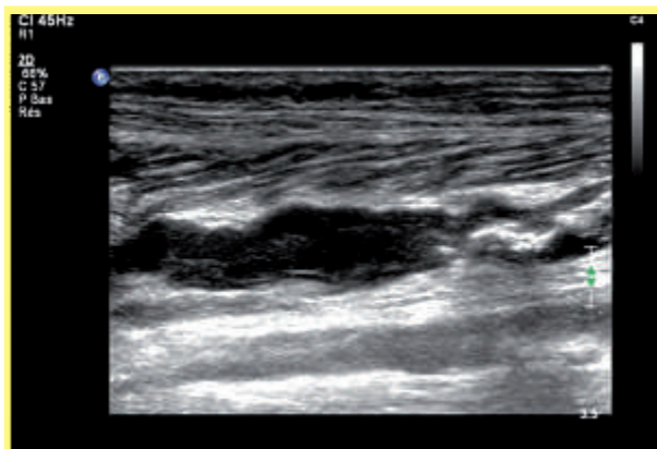
Fig. 19 : Veine fibulaire (coupe longitudinale) : récidue de TVP sur des séquelles fibreuses endoluminales pré existantes.
