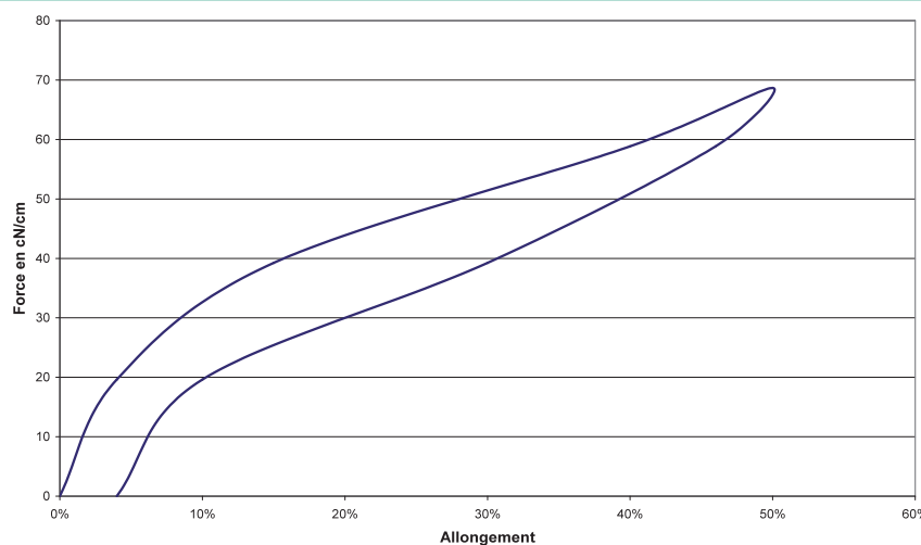
FIGURE 7 : Courbe d'hystérésis d'une bande élastique à allongement long à plat.
