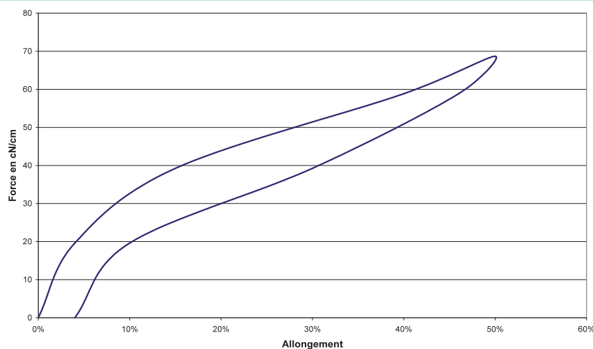
FIGURE 7 : Courbe d'hystérésis d'une bande élastique à allongement court à plat.
